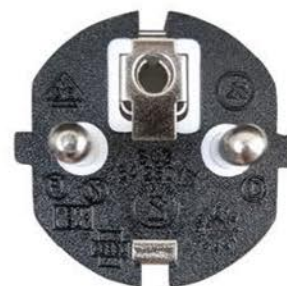
SCHUKO PLUG
